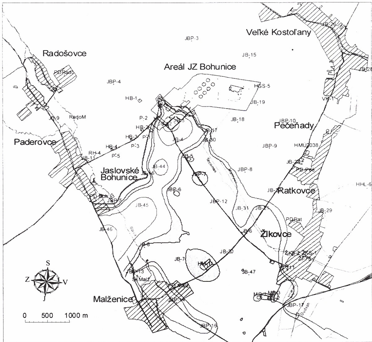
Abb. 6 Isolinien der Volumenaktivität von Tritium im Grundwasser in der weiteren Umgebung území (Stand August 2005)
