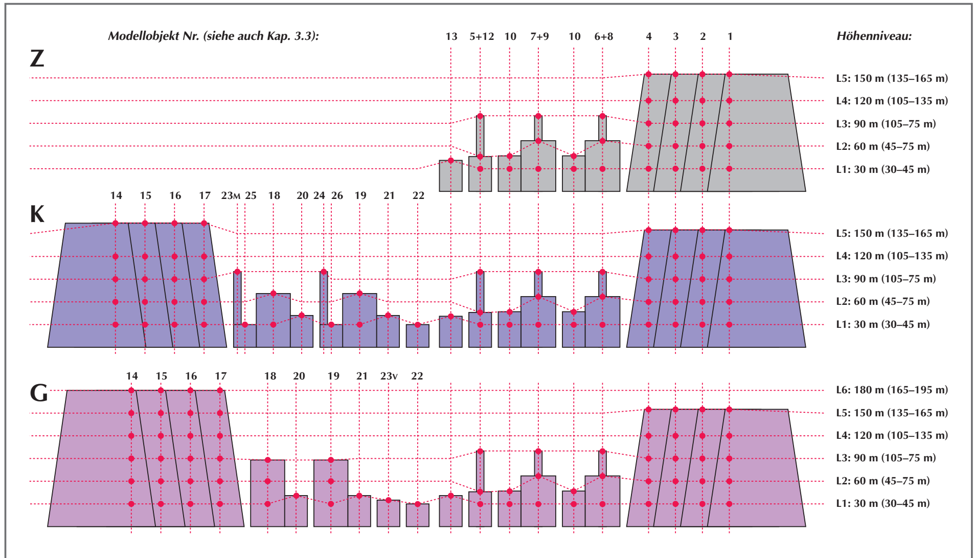
Bild 1: Schematische Darstellung der zu bewertenden Varianten (Z, K und G) und ihrer räumlichen Struktur im verwendeten Sichtbarkeitsmodell des Bauwerkes (siehe Kap. 4.1.1.):
