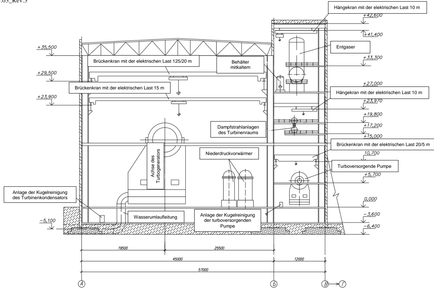
Abbildung 2.12 – Längsquerschnitt des Turbinen- und Entgasungsbereiches
