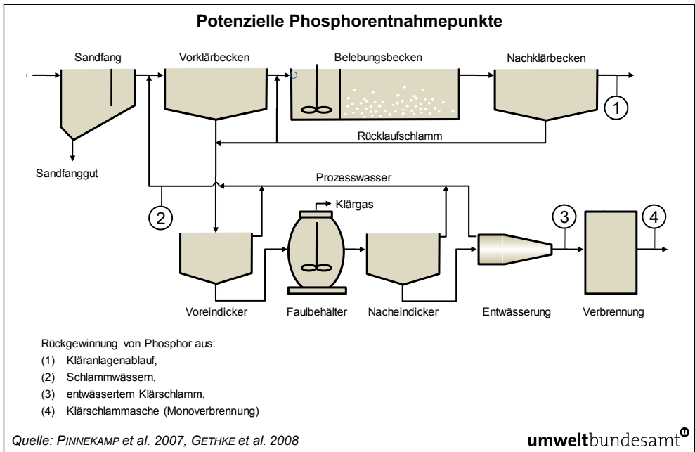
Abbildung 19: Einsatzstellen zur Phosphor-Rückgewinnung auf kommunalen Kläranlagen (PINNEKAMP et al. 2007, GETHKE et al. 2008).
