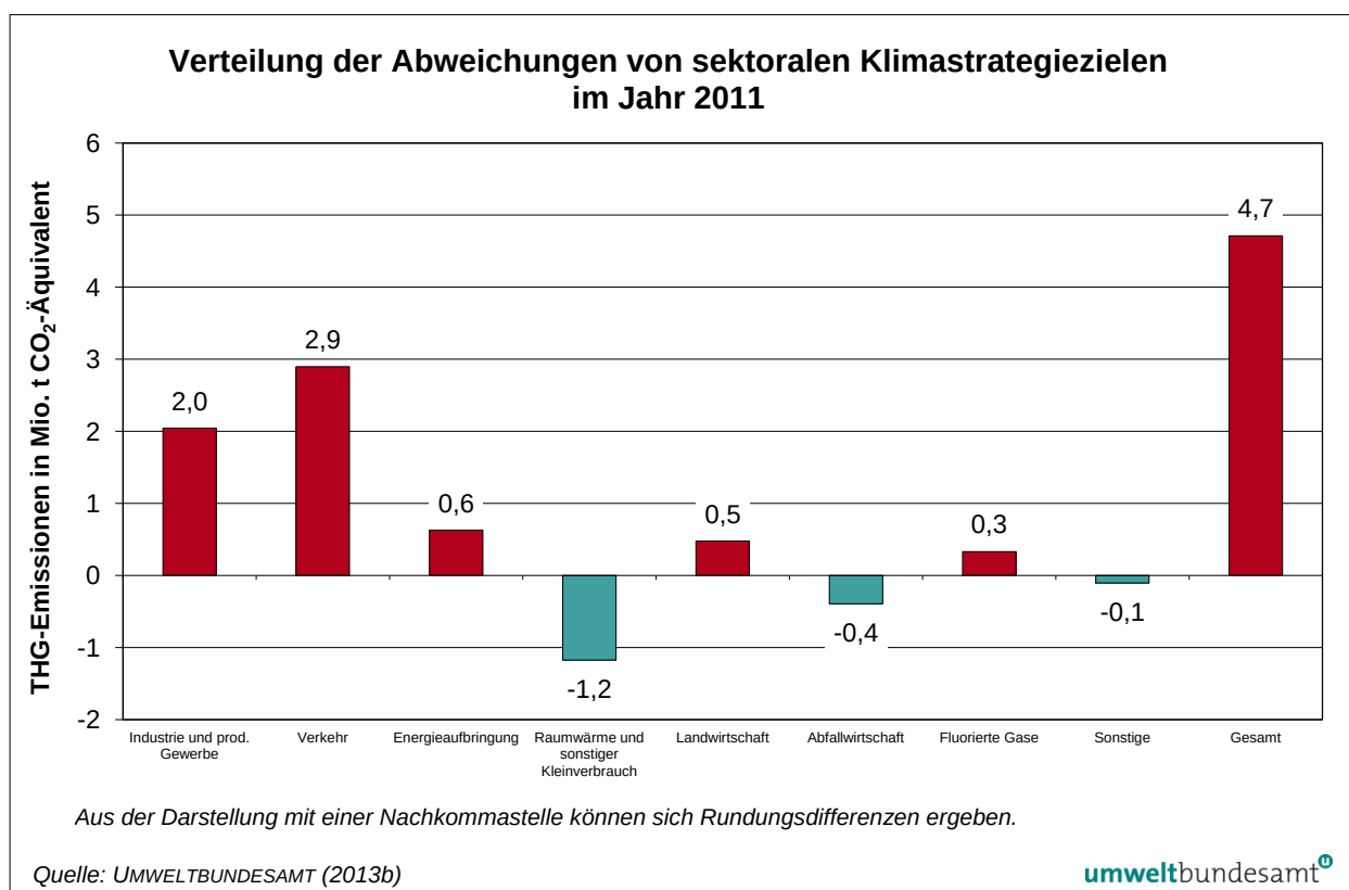
Abbildung 16: Sektoriale Verteilung der Abweichungen vom Ziel der Klimastrategie, 2011. Die Abweichungen der Sektoren Energieaufbringung sowie Industrie und produzierendes Gewerbe beziehen sich ausschließlich auf den Nicht-Emissionshandelsbereich.
