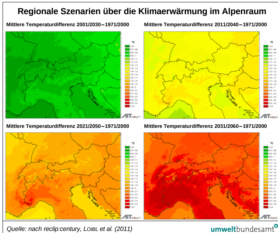
Abbildung 23: Regionale Szenarien über die Klimaerwärmung im Alpenraum, jeweils Differenz von 30-jährigen Mitteln zur Periode 1971–2000, basierend auf dem Modell GCM HADCM3.
