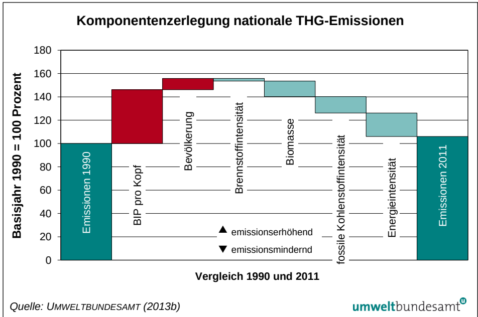
Abbildung 18: Einfluss wichtiger Faktoren auf den Anstieg der Treibhausgas-Emissionen von 1990 auf 2011 (Komponentenzerlegung).
