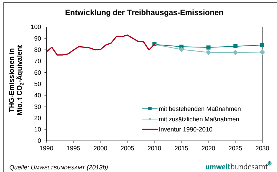
Abbildung 20: Projektion der Treibhausgas-Emissionen Österreichs.
