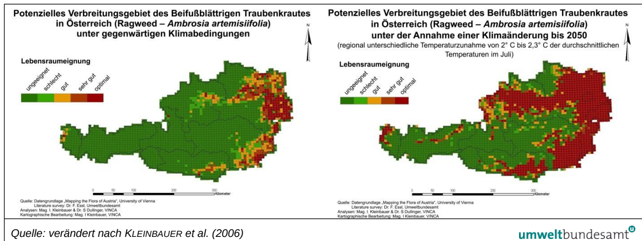
Abbildung 27: Modellierung der Habitateignung der Ambrosie ( Ambrosia artemisiifolia ) in Österreich unter heutigem Klima (a) sowie bei einem Temperaturanstieg von 2,2 °C, wie er für die Mitte des 21. Jahrhunderts möglich ist.
