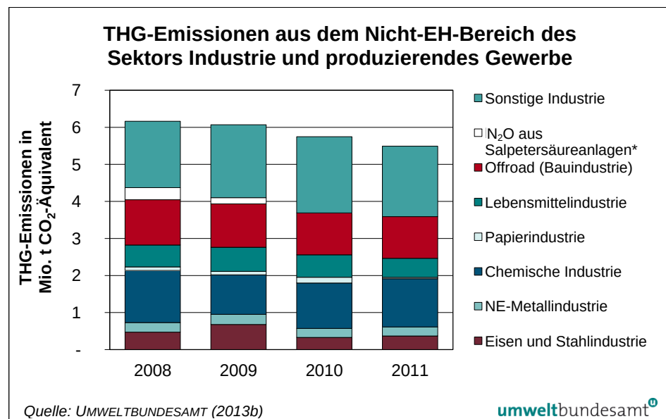
Abbildung 44: Treibhausgas-Emissionen des Sektors Industrie außerhalb des Emissionshandels.
